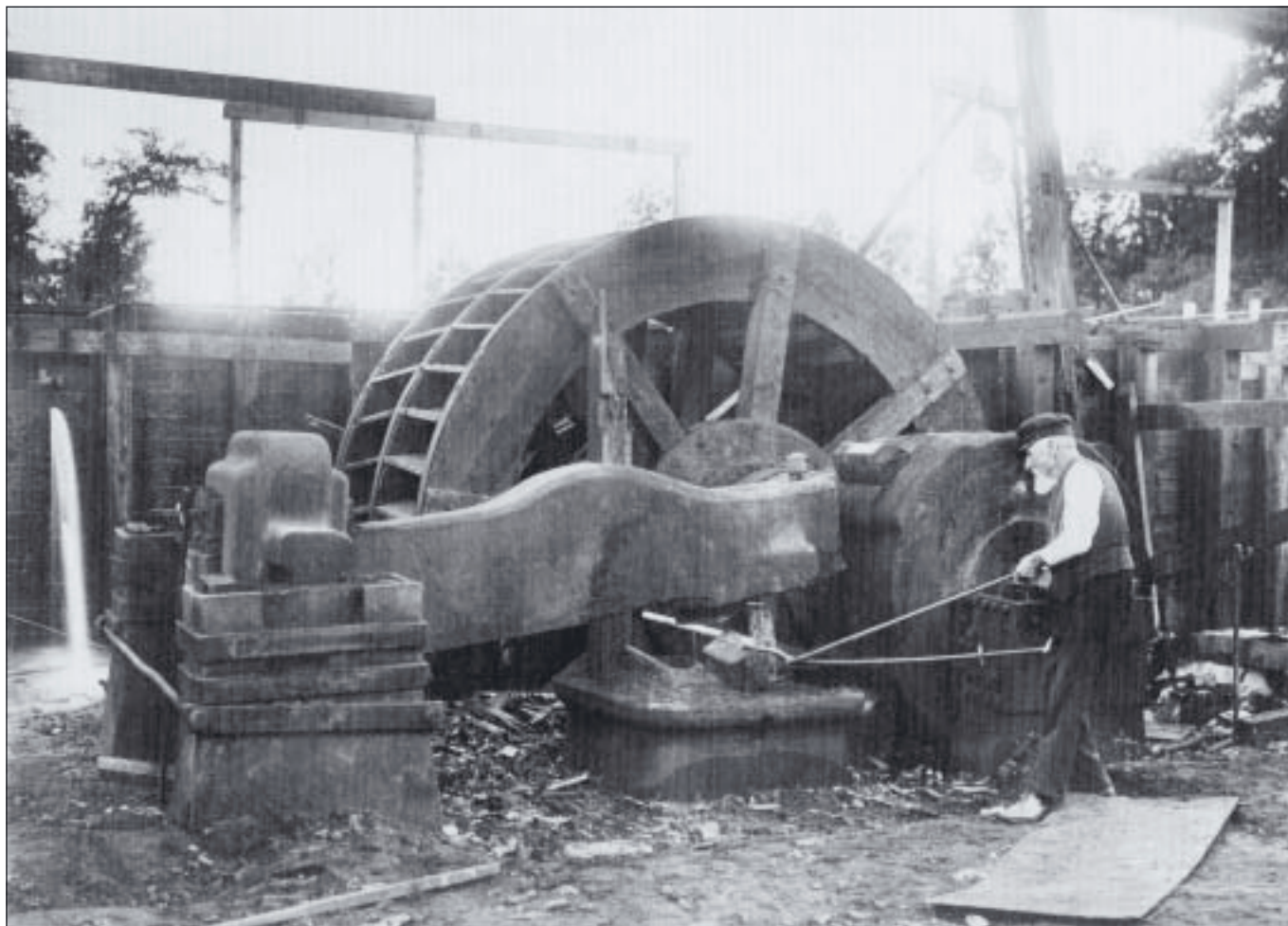
Mumblinghammare vid resterna av Lancarshirsmedjan vid forsen i Bofors. Bilden från år 1918.
